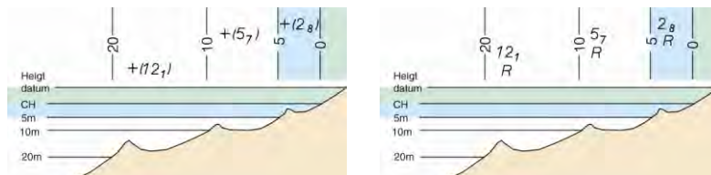
K14.1 Roca peligrosa siempre cubierta de profundidad conocida, dentro de la zona correspondiente a su sonda
