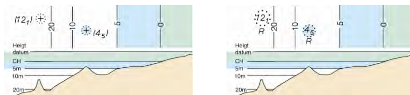
K14.2 Roca peligrosa siempre cubierta de profundidad conocida, fuera de la zona correspondiente a su sonda
